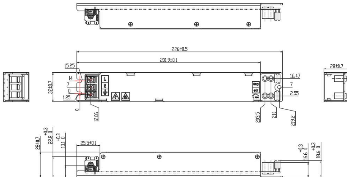
外形尺寸及安装孔——端子坐标
